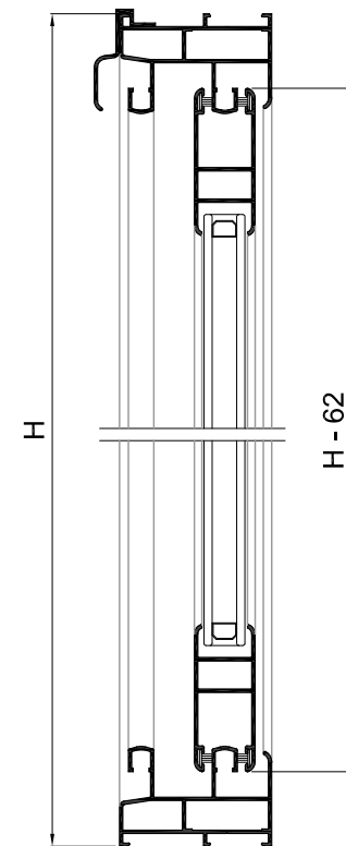
Sección B-B'
