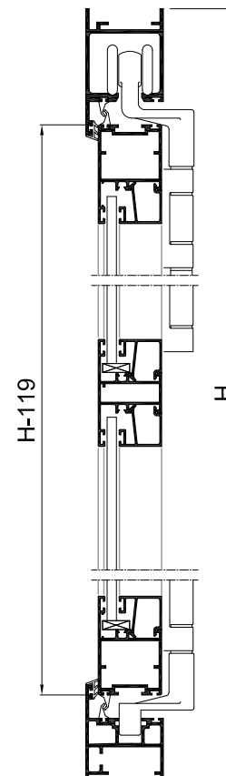
Sección B-B'
