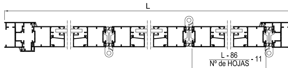
Sección A-A'
